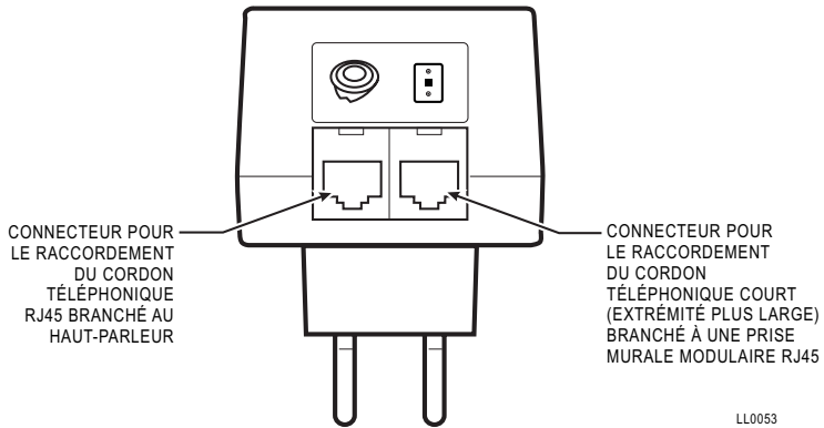
Figure 2 : Adaptateur de courant continu de 48 volts
